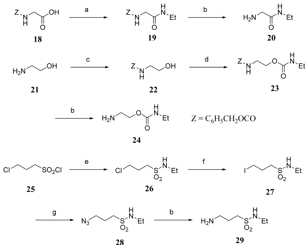
Scheme 4. Preparation of alkylamines possessing an amide moiety. Reagents: (a) EtNH 2 ·HCl, Et 3 N, WSC·HCl, HOBt/THF; (b) H 2 , 10% Pd/C/MeOH; (c) Z-Cl, K 2 CO 3 /H 2 O; (d) EtNCO, pyridine/CH 2 Cl 2 ; (e) EtNH 2 ·HCl, Et 3 N/CH 2 Cl 2 ; (f) NaI/2-butanone; (g) NaN 3 /MeOH-H 2 O.
